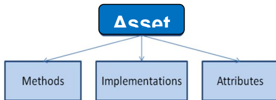
Fig. 3 Assets Meta-model
